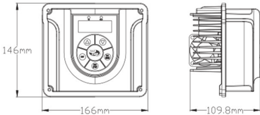
Obrázok 2.1 Rozmery
