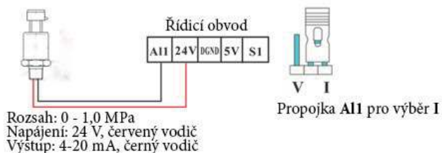
Obrázek 3.2 Snímač tlaku s proudovou zpětnou vazbou
